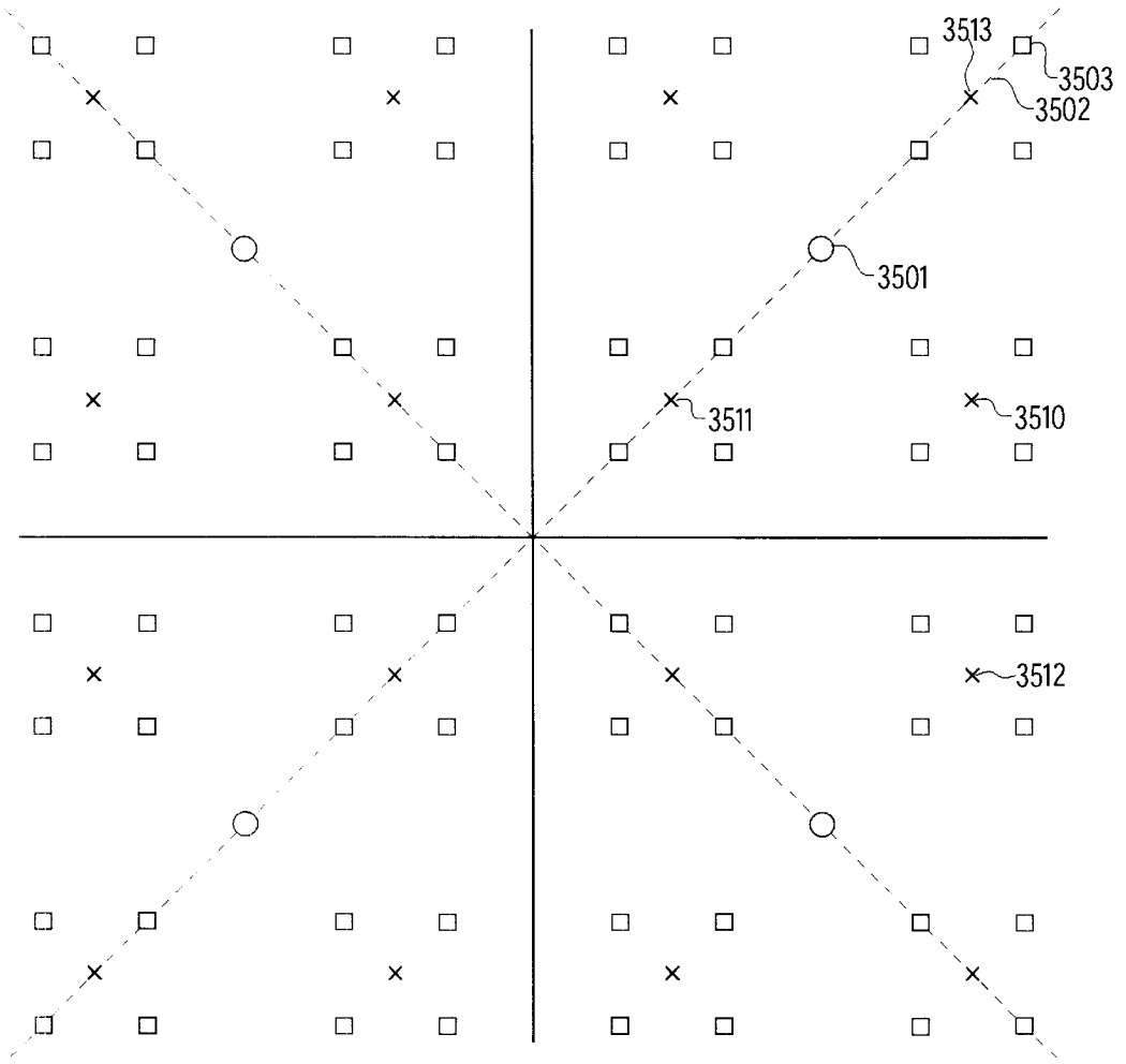
QAM-64
